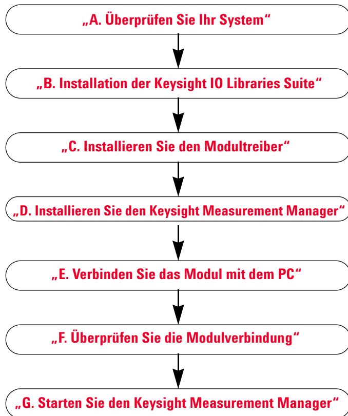
Abbildung 2 Flussdiagramm für Installation und Konfiguration
